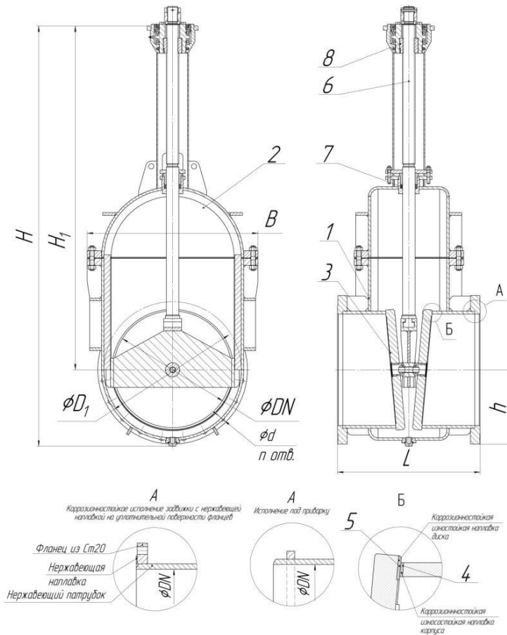
Габаритный чертеж
