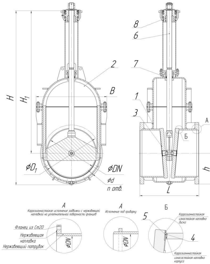
Габаритный чертеж
