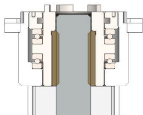
Подшипниковый узел
