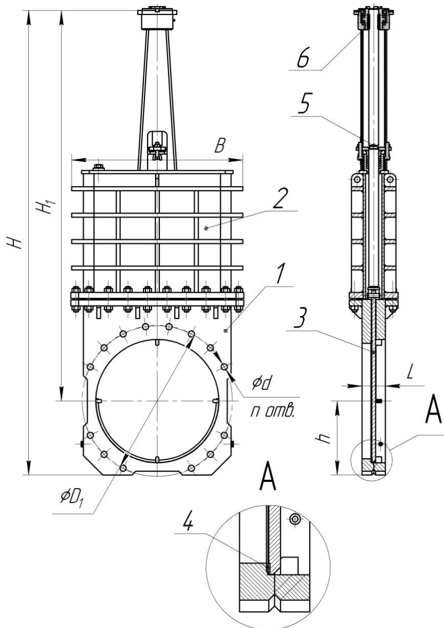
Габаритный чертеж
