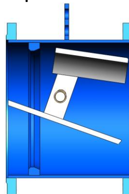
Разрез в положении «Открыто»
