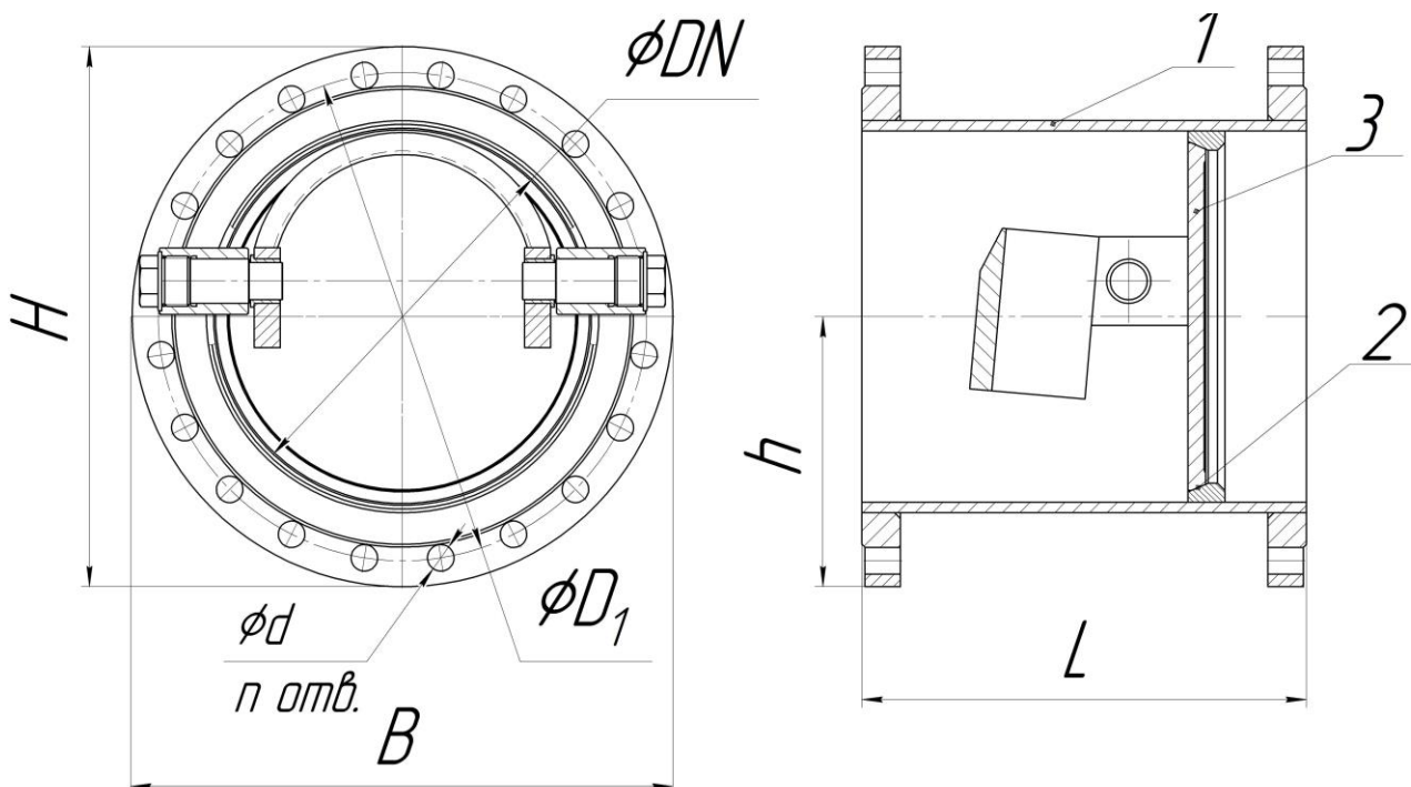
Габаритный чертеж
